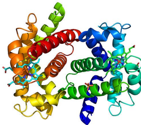
As proteínas dependem de uma dada conformação para serem quimicamente activas.
