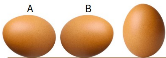
A e B são posições de equilíbrio energético.
