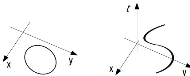
Trajectória de um corpo num plano e a mesma trajectória no espaço (plano) -- tempo. Só a segunda imagem permite conhecer o sentido em que ocorre o movimento.
