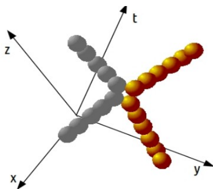
Choque de duas partículas no espaço-tempo.
