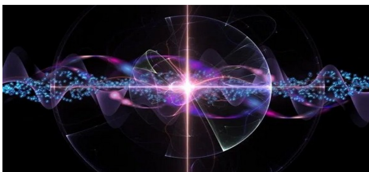
Representação artística de um pequeno fragmento da molécula de ADN.
