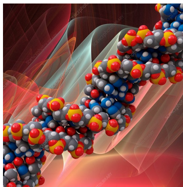
Modelo de um curtíssimo fragmento de uma molécula de ADN.
