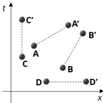
Um universo de quatro partículas
