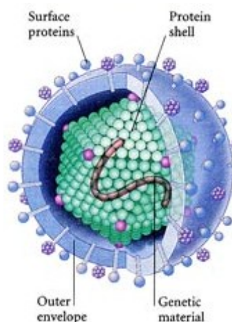
Estrutura de um vírus.
