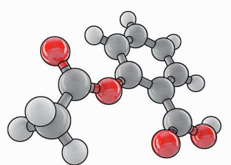
Modelo da molécula da aspirina.
